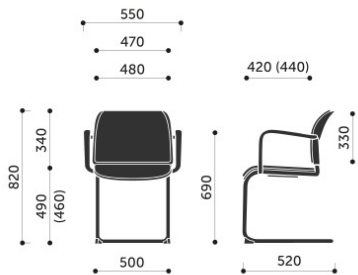
570V / 570V 2P
